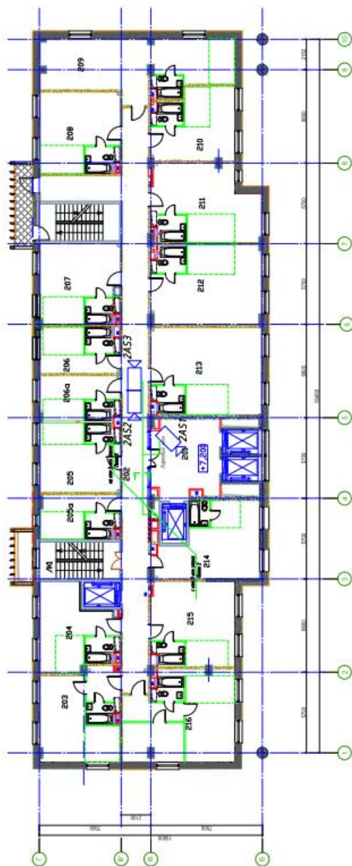
План 2-го этажа в/отм. +7,200
