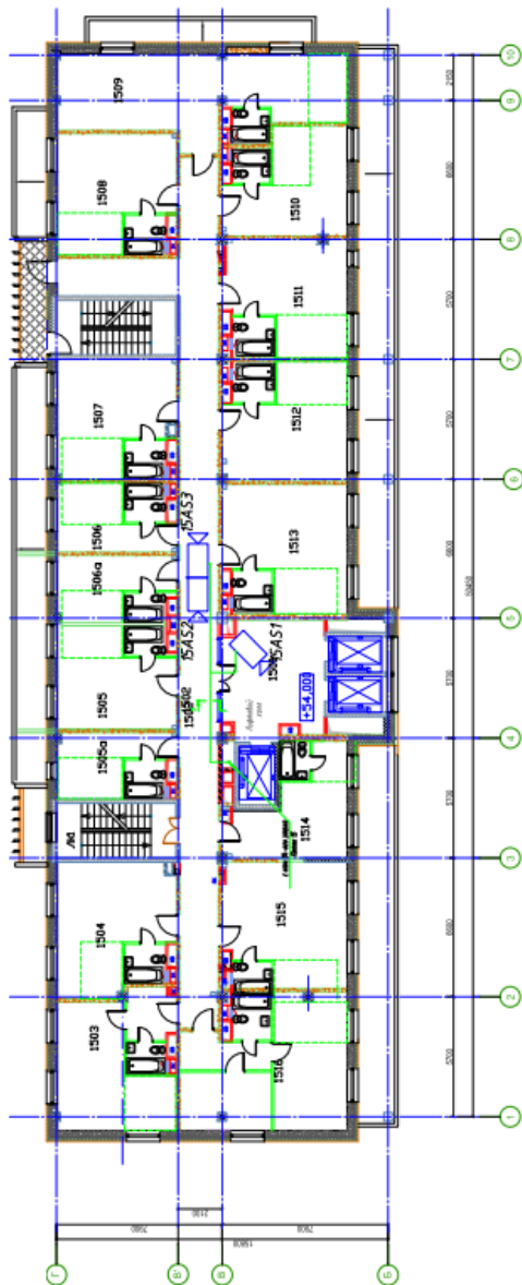
План 15-го этажа
