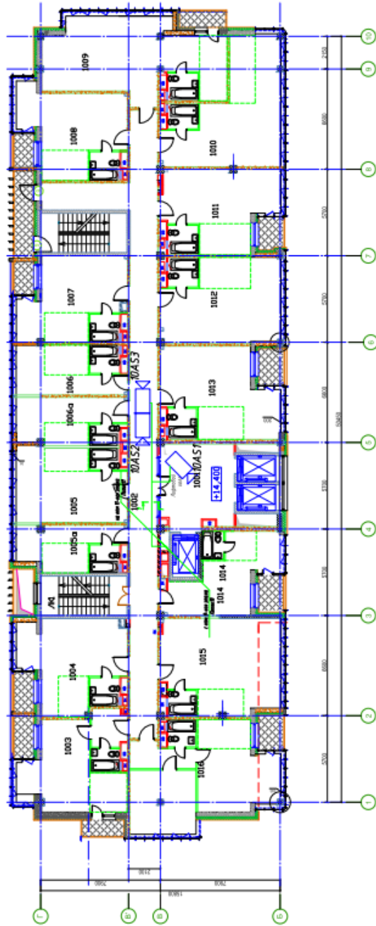
План 10-го этажа
